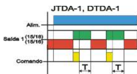
Diagrama de ligação - 10
